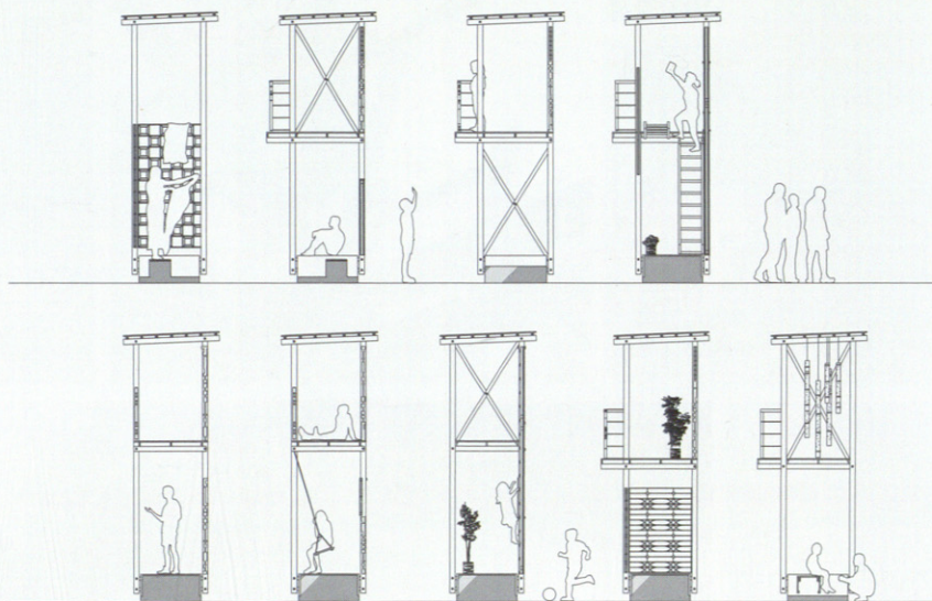
SECCIONES TRANSVERSALES. CROSS SECTIONS.
